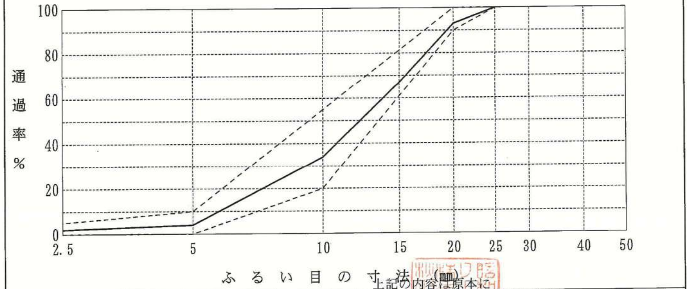
粒 度 曲 線
