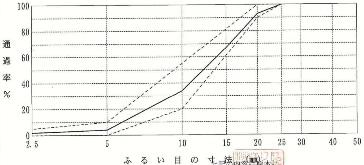
粒 度 曲 線
